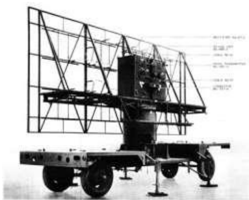
Foto nr. 1, radarul american S.C.R.-527 A
